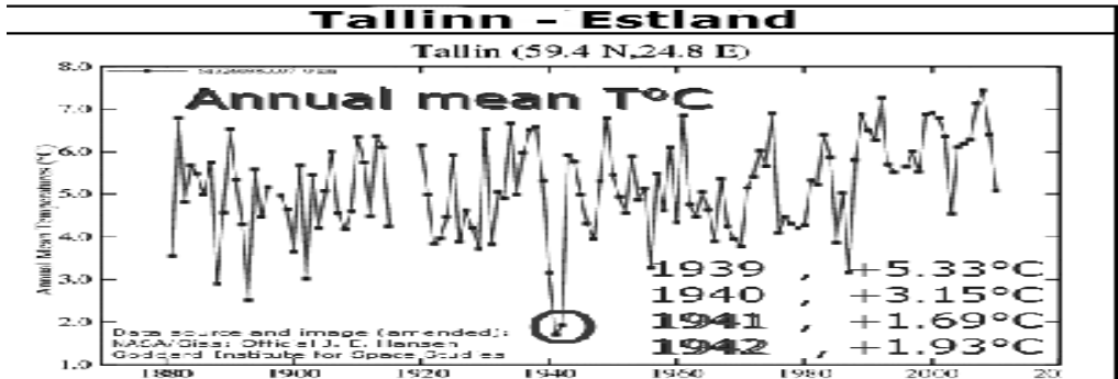
Abb. E3-5; Mittlere Jahrestemperaturen, 1880-2005
